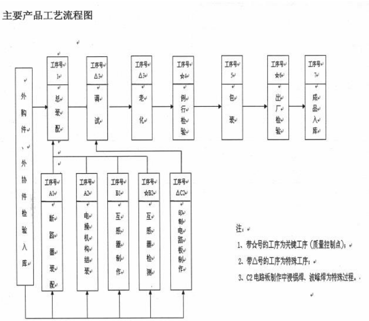
图 3-2 受核查方工艺流程图
