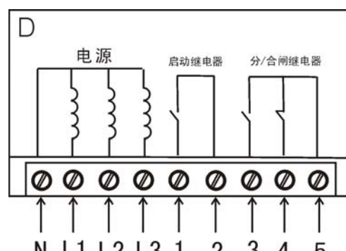
增强 T 型接线桩示意图
