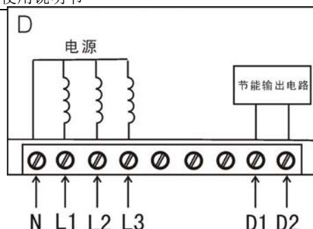
增强 J 型接线桩示意图
